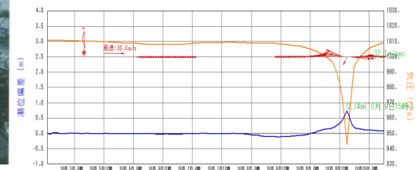
潮位偏差時刻歴
