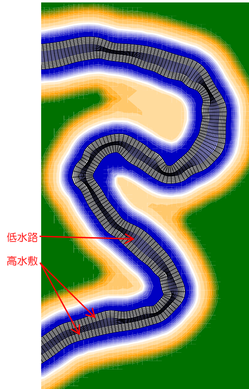
河道のメッシュ作成例 (直交曲線)
