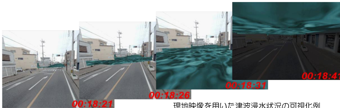
現地映像を用いた3次元災害リスク可視化技術手法の概要
